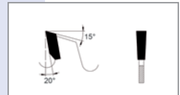
Abb.: Flachzahn (F)
